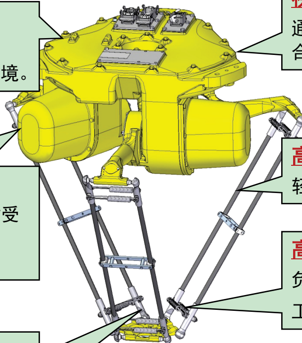
M-3iA/12H
