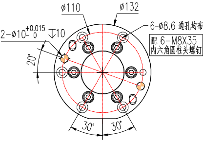
工具本体侧安装尺寸图
