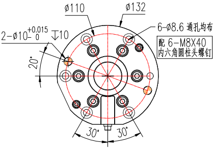
机器人本体侧安装尺寸图
